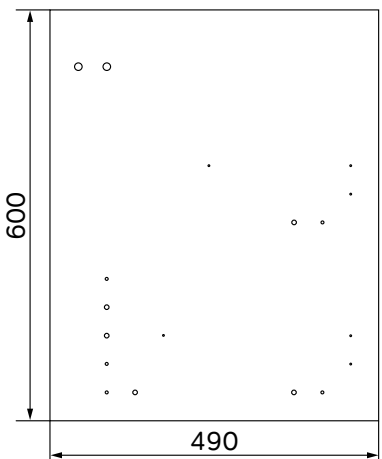
2-Бок правый
