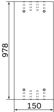
4- Перемичка
