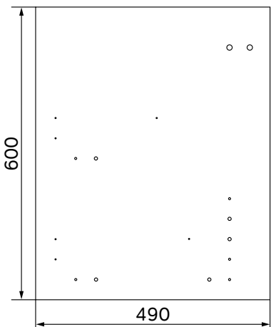
1-Бок левый
