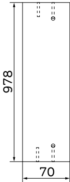
5-Перемичка
